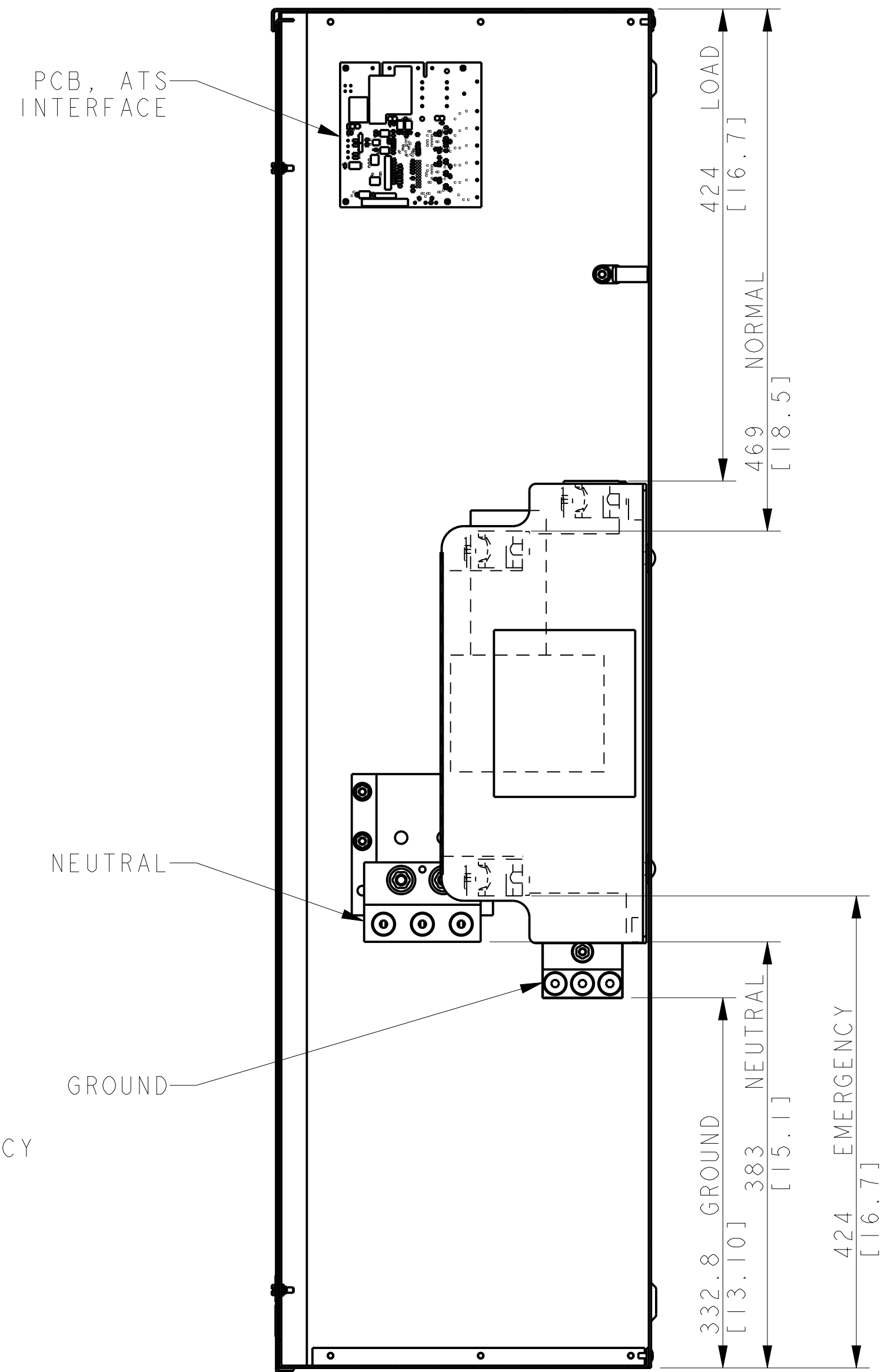
SECTION A-A
