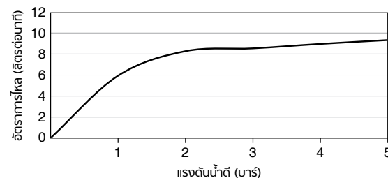
กราฟแสดงการไหล ฝักบัวสายอ่อน
