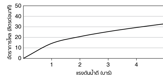
กราฟแสดงการไหล ก๊อกลงอ่าง
