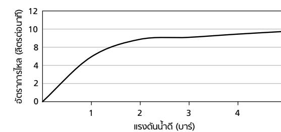
กราฟแสดงการไหลของน้ำ K-28693T
