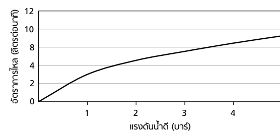
กราฟแสดงการไหลของน้ำ K-28692T
